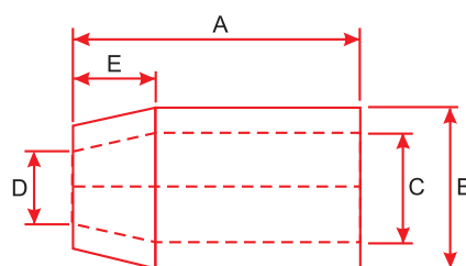
Стальные обжимные втулки B902
